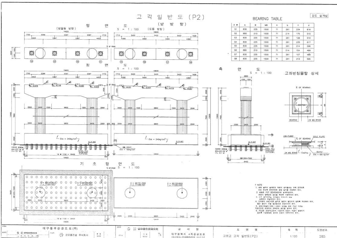
[일반도(교각)]
